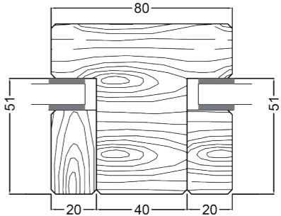
Traverse intermédiaire / Meneau
