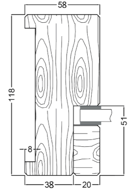
Profil rainuré à brique
